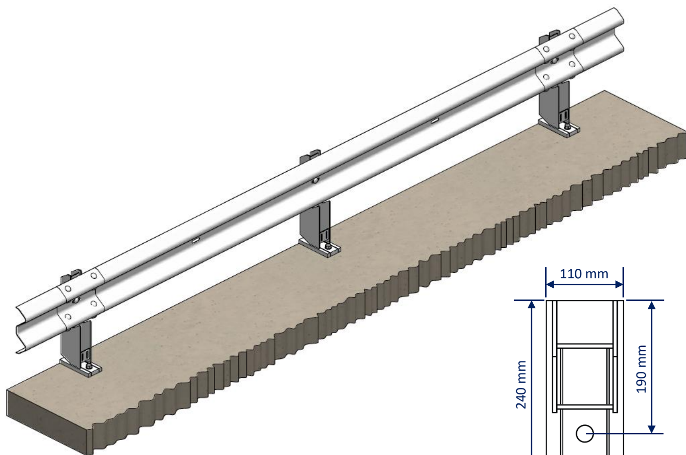
BASEPLATE
